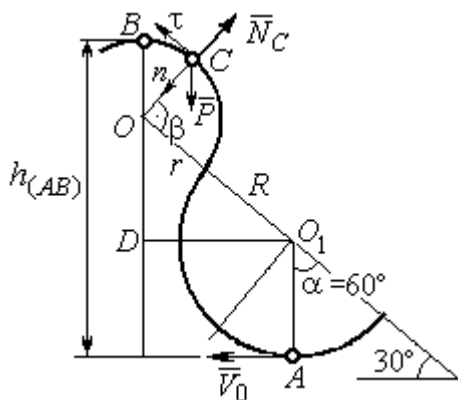
Рис. 4.21. Расчётная схема движения шарика
