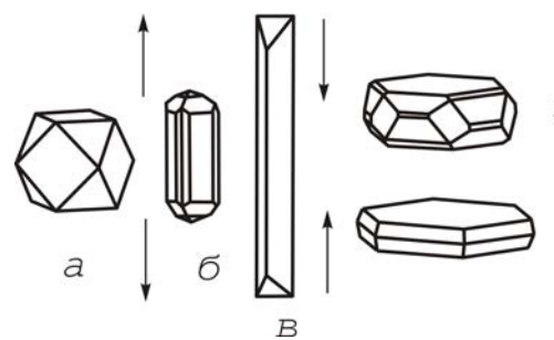
Рис. 3. Типы облика кристаллов: a – изометричный; б – короткопризматический; в – длиннопризматический; г – таблитчатый; д – пластинчатый.
