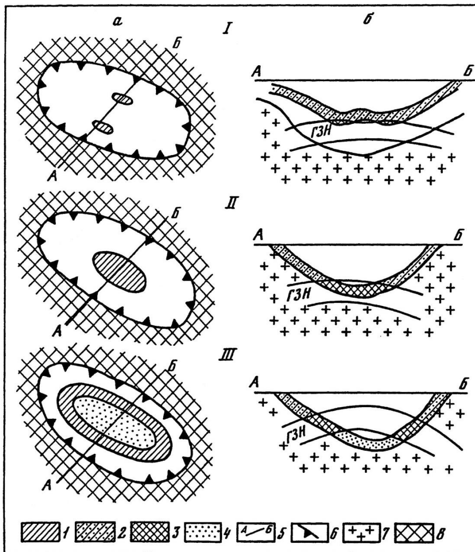
Рис. 13. Типы очагов нефтегазообразования ( а – плановое положение очага в бассейне, б – положение очага в разрезе бассейна) [16]:
