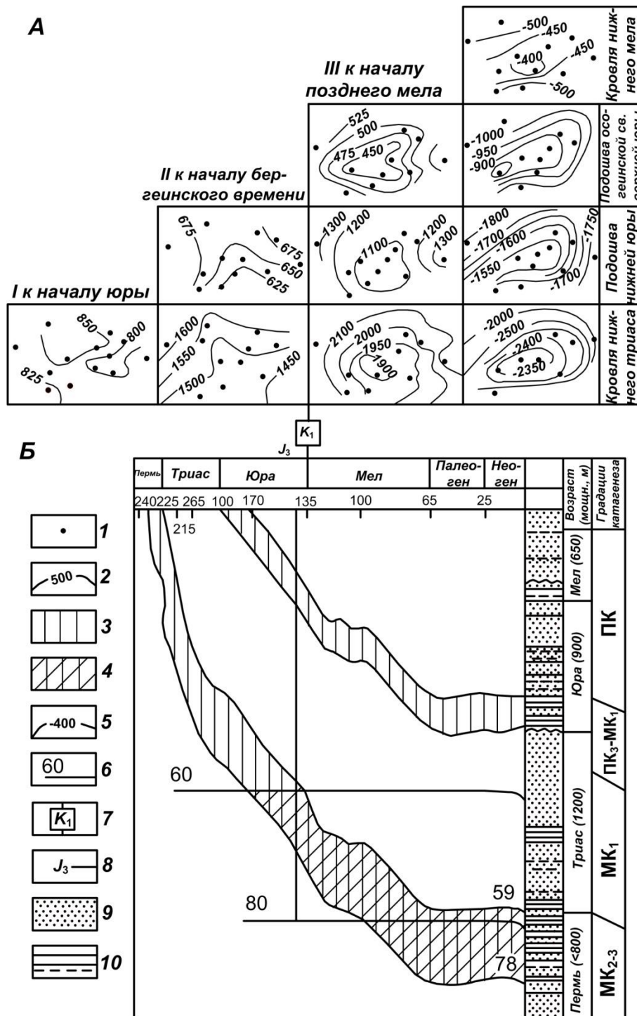
Рис. 5. Генерационно-аккумулятивный хроно-блок. Средне-Вилноийское месторождение (Соколов, Ларченков, 1978):
