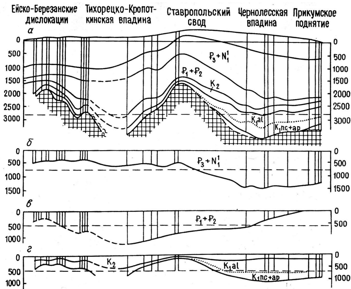
Рис. 1. Современный и палеотектонические профили (профили компенсации) Предкавказья (по Ю. А. Сударикову [2, 3]): a – современный профиль; палеотектонические профили: б – к началу среднего миоцена (мощность майкопской серии), в – к началу майкопского времени (мощность палеоцена и эоцена), г – к началу палеогена (мощность мела)
