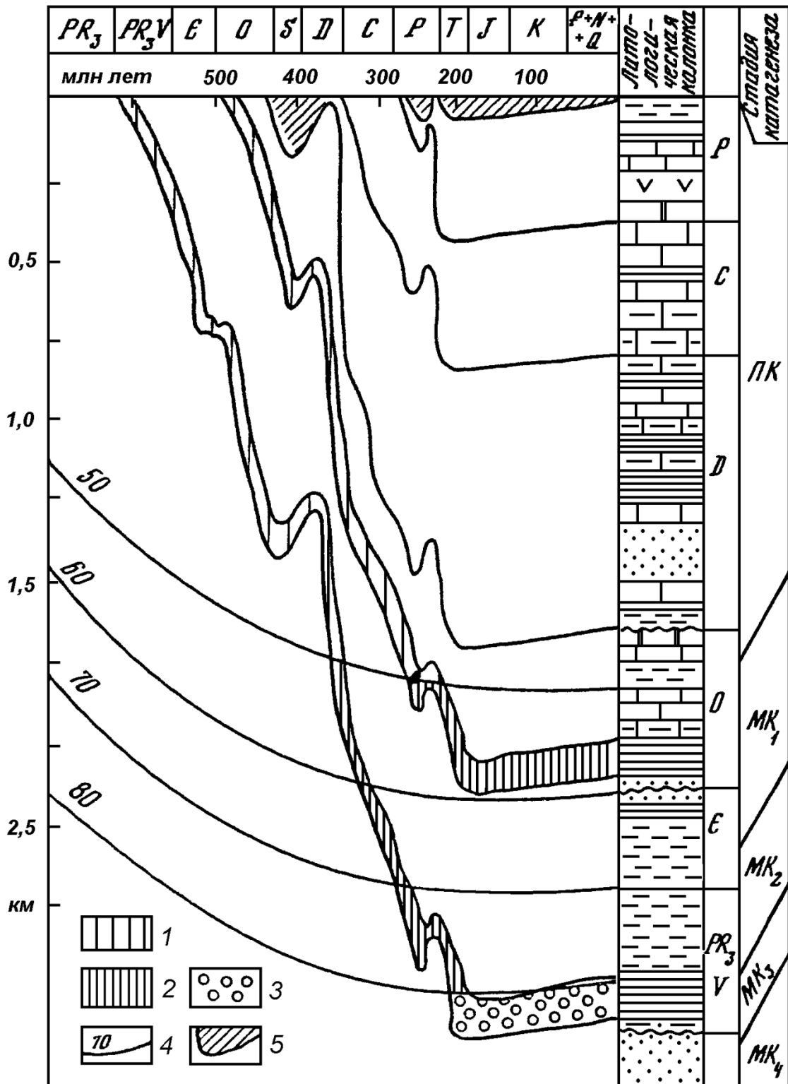
Рис. 11. Модель прогрева отложений для Любимской площади (Среднерусский бассейн) [16]: отложения: 1 – нефтематеринские, 2 – нефтепроизводящие, 3 – нефтепроизводившие, 4 – изотермы (°C); 5 – перерывы в осадконакоплении; в литологической колонке показано переслаивание известняков, мергелей, глин, аргиллитов и песчаников
