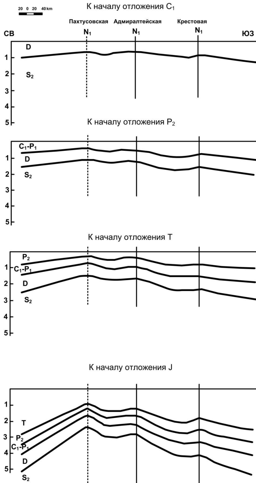
Рис. 3. Палеотектонические профили через Адмиралтейский вал [17]
