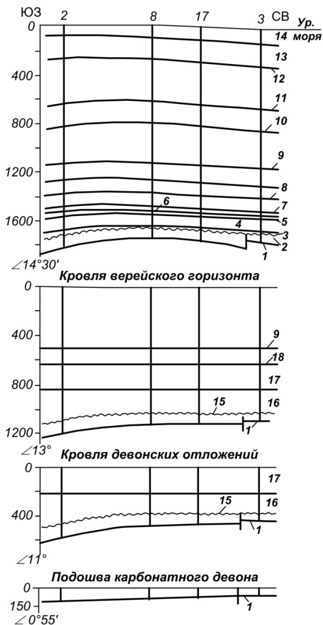
Рис. 2. Современный и палеотектонические профили вкрест простирания Генеральского поднятия (Саратовское Поволжье) [1]:
