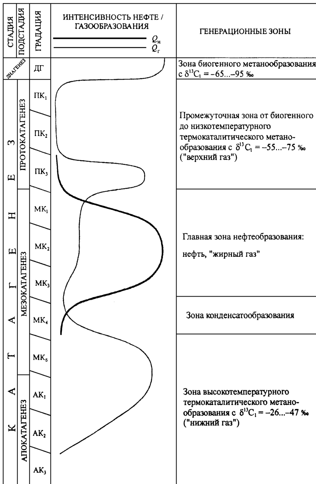
Рис. 9. Обобщенная традиционная схема вертикальной зональности нафтидогенеза (заимствовано из работы Е. И. Тараненко и др. «Современные аспекты вертикальной зональности нафтидогенеза», 2008)
