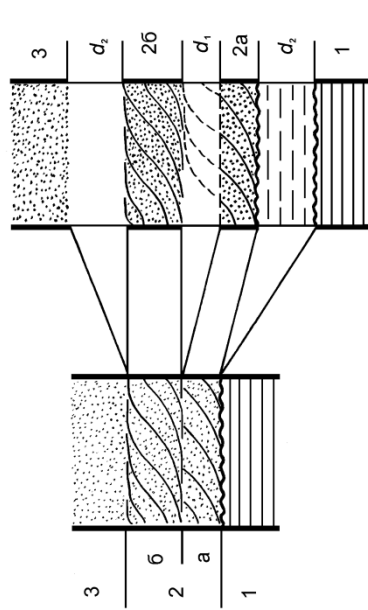
Рис. 6.4. Схематическое изображение соотношения слоев и разделяющих их перерывов (диаستم):
