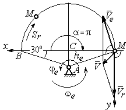
Рис. 3.8. Расчетная схема для вычисления абсолютной скорости точки
