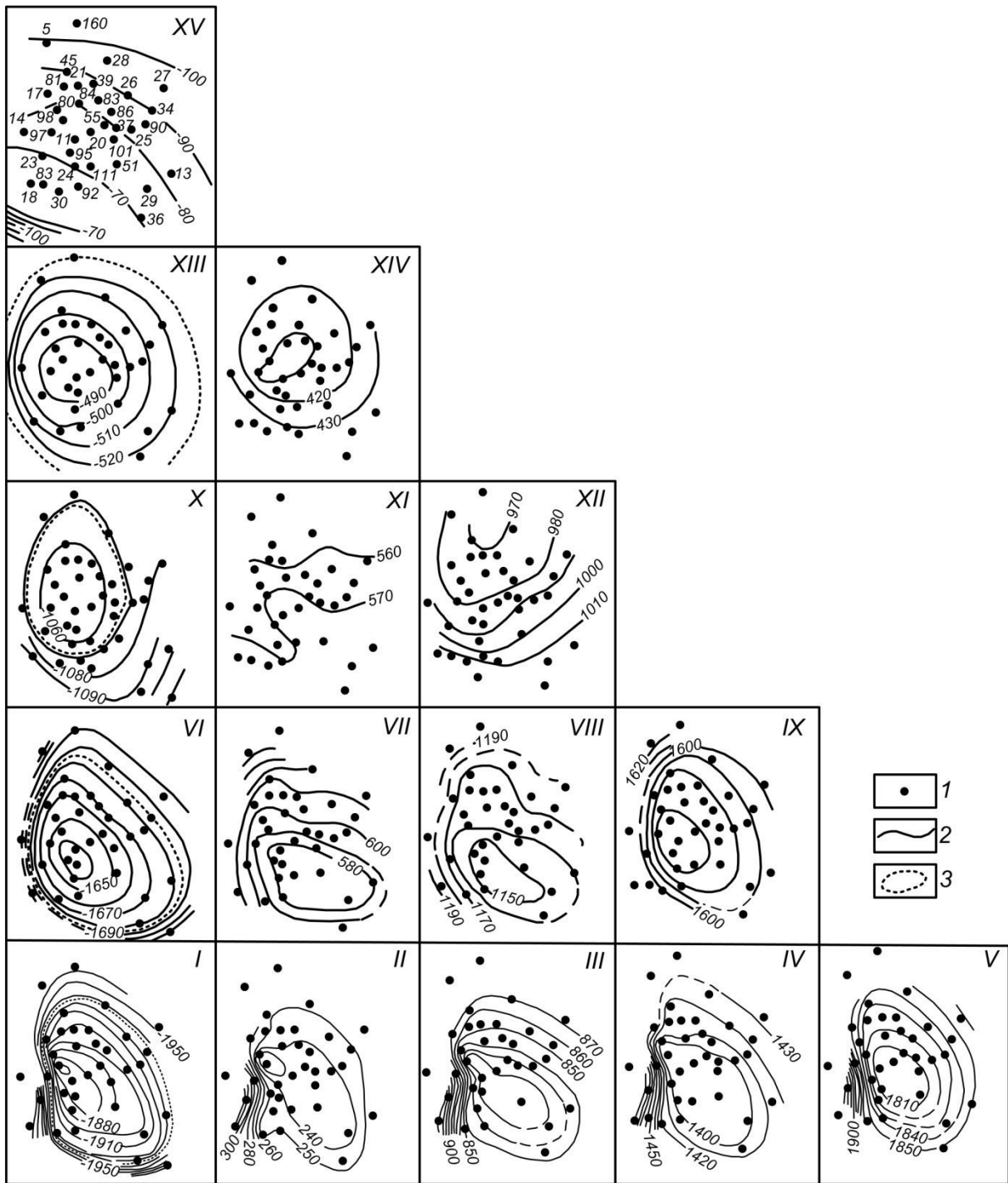
Рис. 6. Структурные и палеоструктурные карты Соколовогорского поднятия [1]: 1 – скважины; 2 – изогипсы и изопахиты; 3 – контуры нефтяных и газовых залежей
