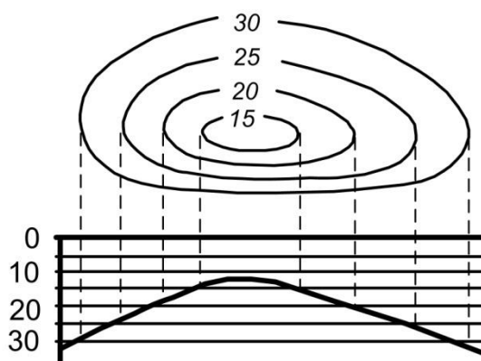
Рис. 4. Схема расположения карт в изопактическом треугольнике и принцип построения палеоструктурных карт [2]
