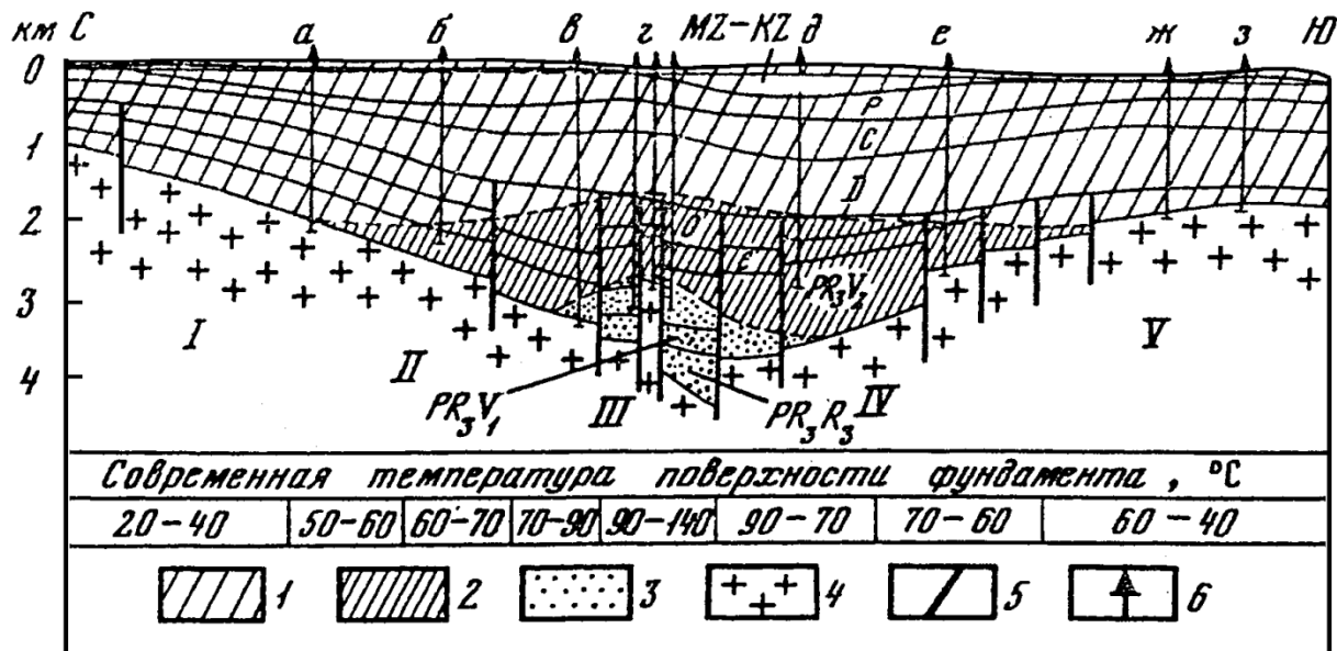
Рис. 12. Схема положения зон генерации УВ Среднерусского бассейна (составили Б. А. Соколов, В. А. Егоров, Ю. И. Корчагина) [16]:
