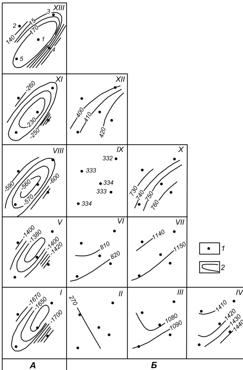
Рис. 7. Структурные и палеоструктурные карты Гусихинского поднятия [1]: А – структурные карты: I – по кровле пласта D_2-V ; V – по подошве карбонатных девонских отложений; VIII – по кровле тульского горизонта ( C_{1v2} ); XI – по кровле верейского горизонта ( C_{2m} ); XIII – по кровле барремского яруса; Б – палеоструктурные карты: II – кровля пласта D_2-V ; к началу отложения карбонатного девона; кровля пласта D_2-V к концу; III – тульского и IV – верейского времени; подошва карбонатных девонских отложений к концу: VI – тульского и VII – верейского времени; кровля тульского, горизонта к концу: IX – верейского времени и X – барремского века; XII – кровля верейского горизонта к концу барремского века; 1 – скважины; 2 – изогипсы и изопахиты
