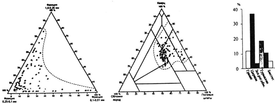
Рис. 8.2. Гранулометрический, вещественный и минералогический состав пород пласта ЮС 1 3 аллювиально-дельтового комплекса. Среднеvasюганский мегавал (Л. С. Чернова и др., 2004)
