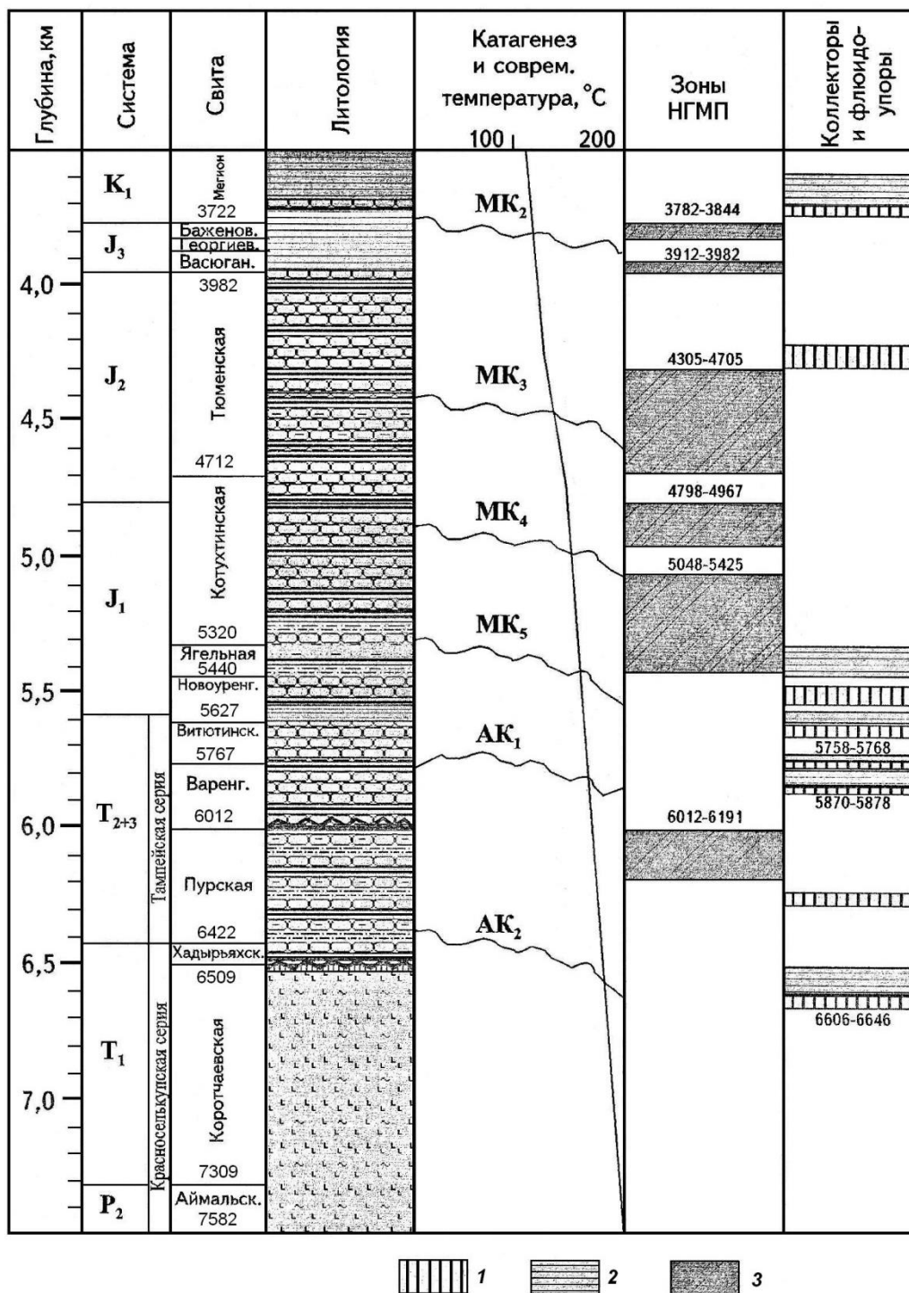
Рис. 16. Схематический геологический разрез СГ-6 (Т. В.Белоконь-Карасева, 2006): 1 – коллекторы; 2 – флюидоупоры; 3 – нефтегазоматеринские породы
