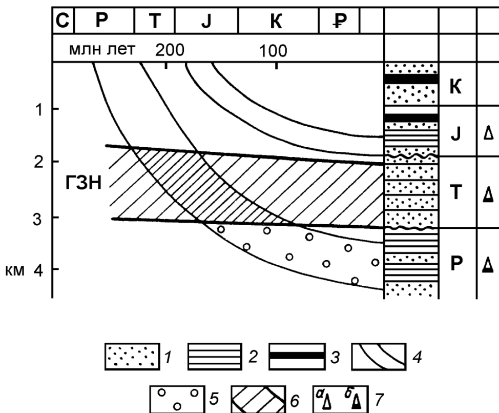
Рис. 10. Принцип построения-модели прогрева (Соколов, Ларченков, 1985): 1 – песчаники; 2 – глины; 3 – каменный уголь; 4 – нефтематеринские породы; 5 – газопроизводящие породы; 6 – ГЗН; 7 – залежи: а – газовые, б – нефтяные и нефтегазовые
